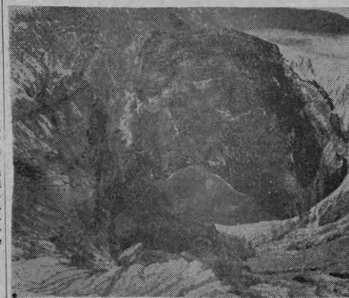
En la fotografía se aprecia la chimenea principal del cráter del Irazú con su laguna de aguas color pardo-rojizo. Esta chimenea es la que está atascada y la que cualquier día puede hacer explosión.
